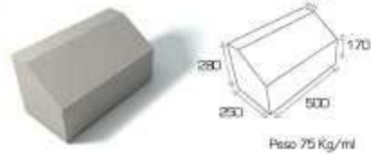
Pieza central
